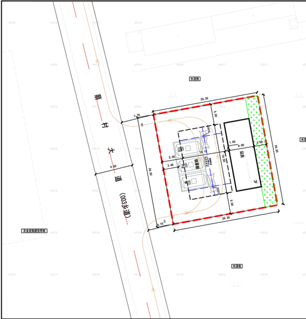
总平面布置示意图
