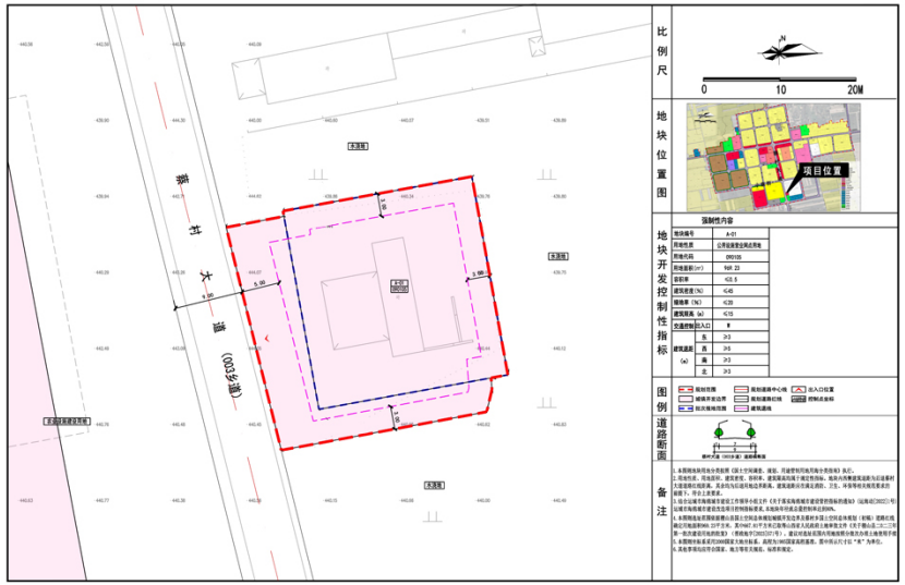
总平面布置示意图
